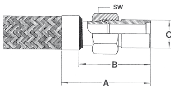
7C. wie Abb. 7, aber Einschraubteil mit Anschweißrohrstutzen
